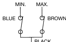
LMM1GSA MIN. - MAX. CONTACTS
