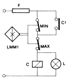
Riempimento automatico Automatic filling
