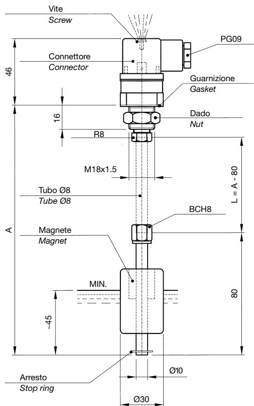
Schema di applicazione Application chart
