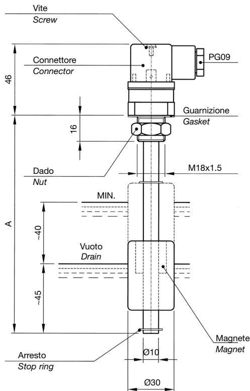
Schema di applicazione Application chart
